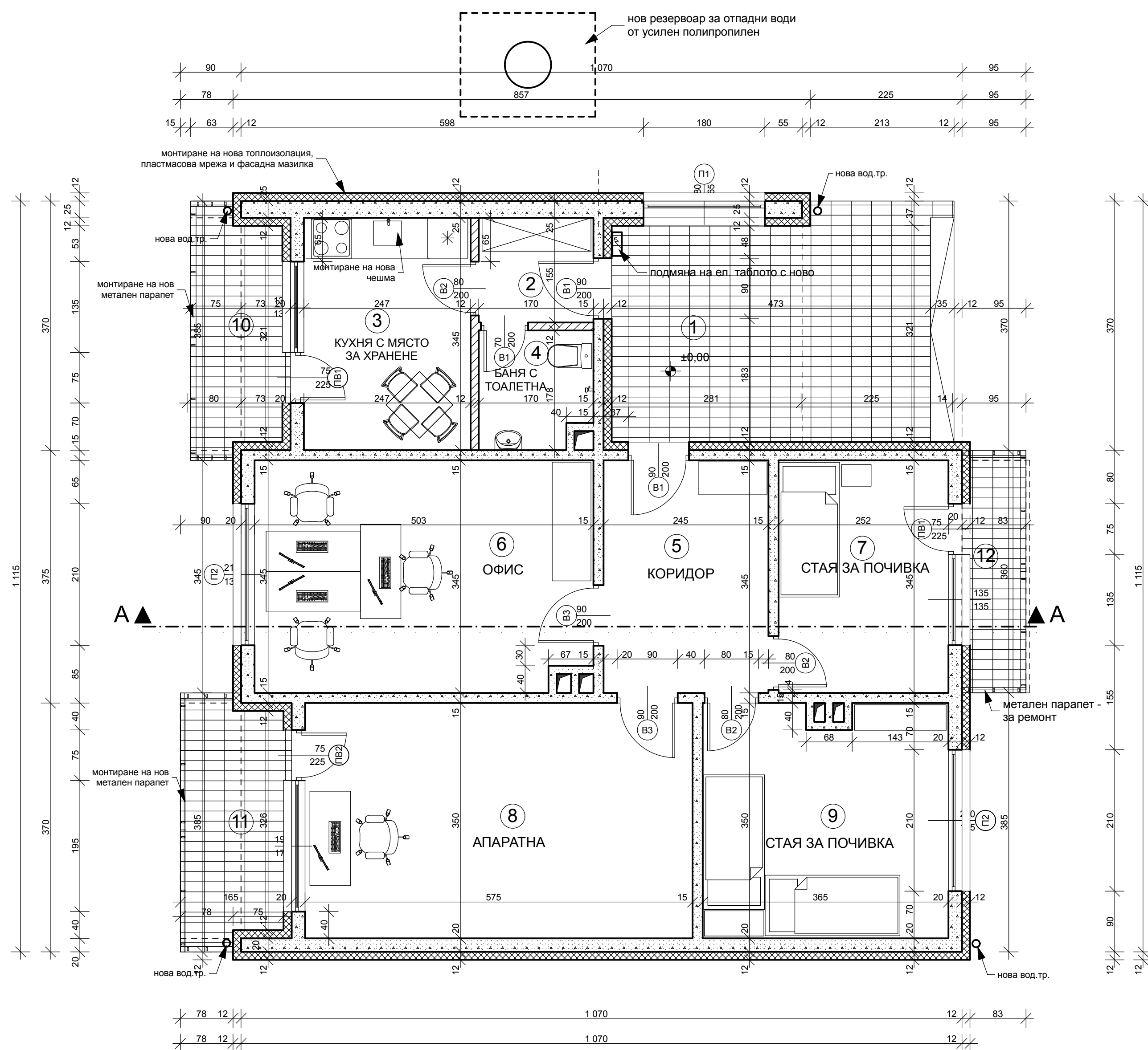
РАЗПРЕДЕЛЕНИЕ на ката ±0,00
